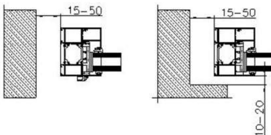
Рисунок 4.2 - Размеры монтажных зазоров (швов) при установке алюминиевых конструкций
