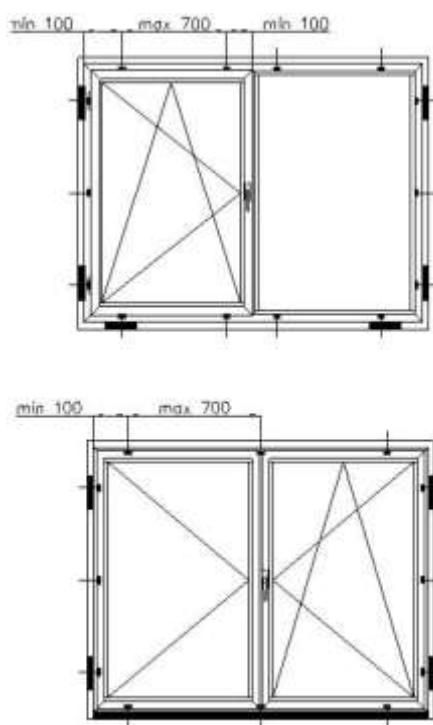
Рисунок 4.3 - Примеры расположения опорных (несущих) колодок и крепежных деталей при установке оконных блоков
