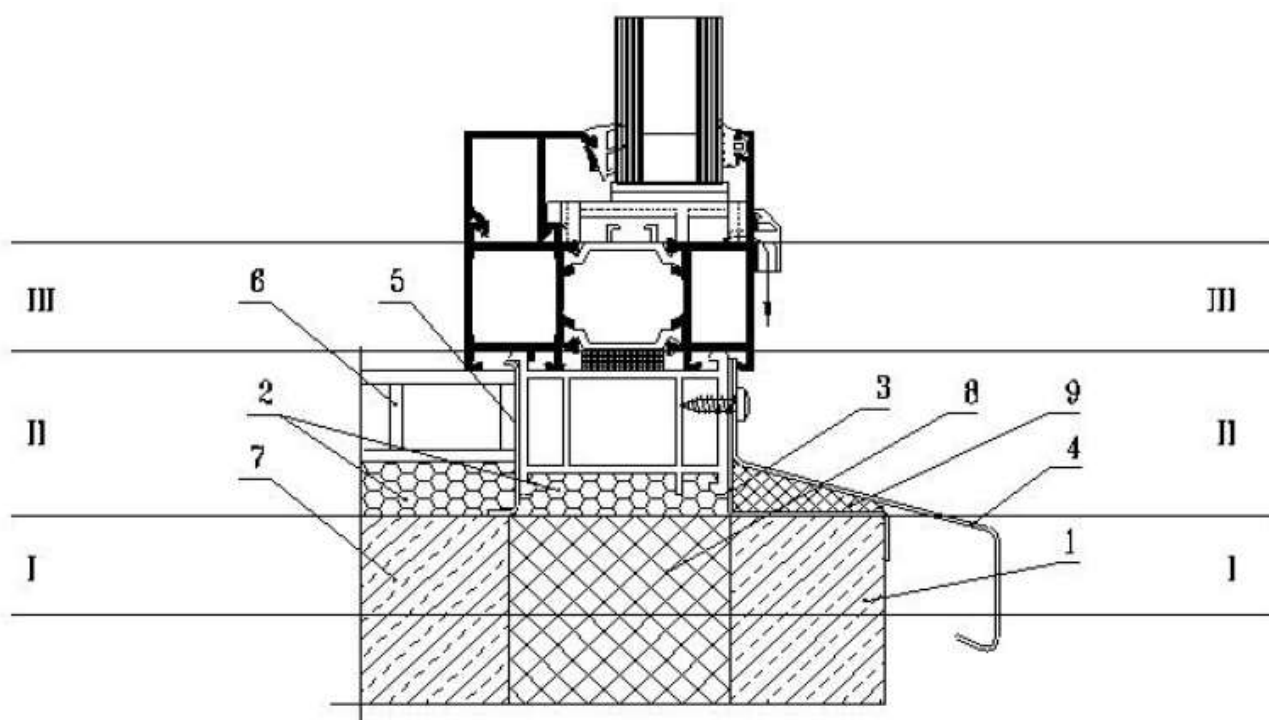
Рисунок 4.1- Узел примыкания алюминиевой конструкции к проему многослойной стены (возможный вариант).
