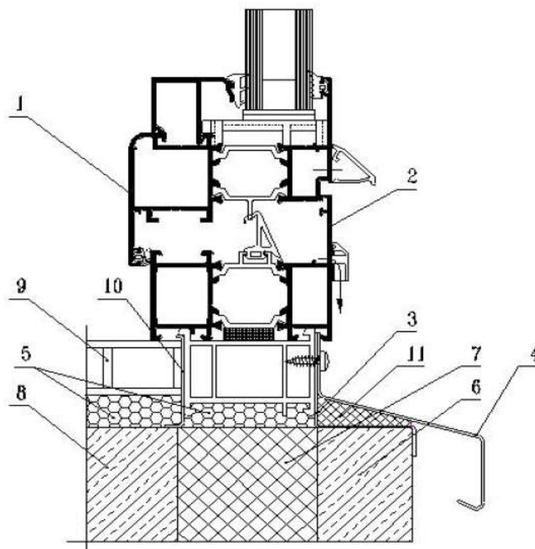
Рисунок А.1 - Узел примыкания алюминиевого оконного блока к проему слоистой кирпичной стене с отделкой наружных и внутренних откосов штукатурным раствором.
