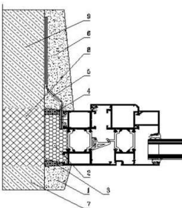
Рисунок А.2 - Узел примыкания оконного блока к стеновому проему без четверти слоистой кирпичной стены
