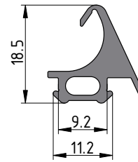
ТПУ-6005 (M=0.02кг/м)
