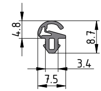
ТПУ-006-01ММ (M=0.031кг/м)
