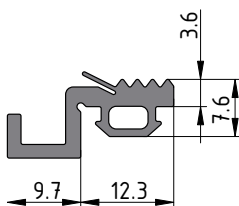
ТПУ-6001К (M=0.110кг/м)
