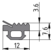
ТПУ-6001 (M=0.066кг/м)
