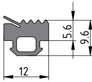
ТПУ-001ММ (M=0.075кг/м)
