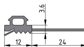
ТПУ-6001Т (M=0.11кг/м)
