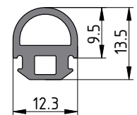
ТПУ-6010 (M=0.1кг/м)
