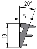
ТПУ-004ММ (M=0.055кг/м)
