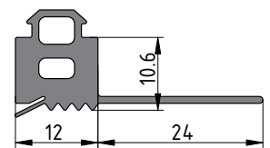
ТПУ-6002Т (M=0.19кг/м)
