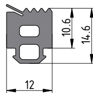
ТПУ-6002 (M=0.140кг/м)
