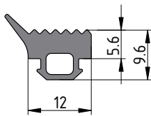
ТПУ-007ММ (M=0.085кг/м)
