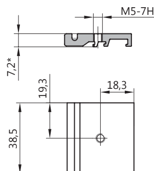
СОЕДИНИТЕЛЬ ИМПОСТА ТПТ-65.08.01
