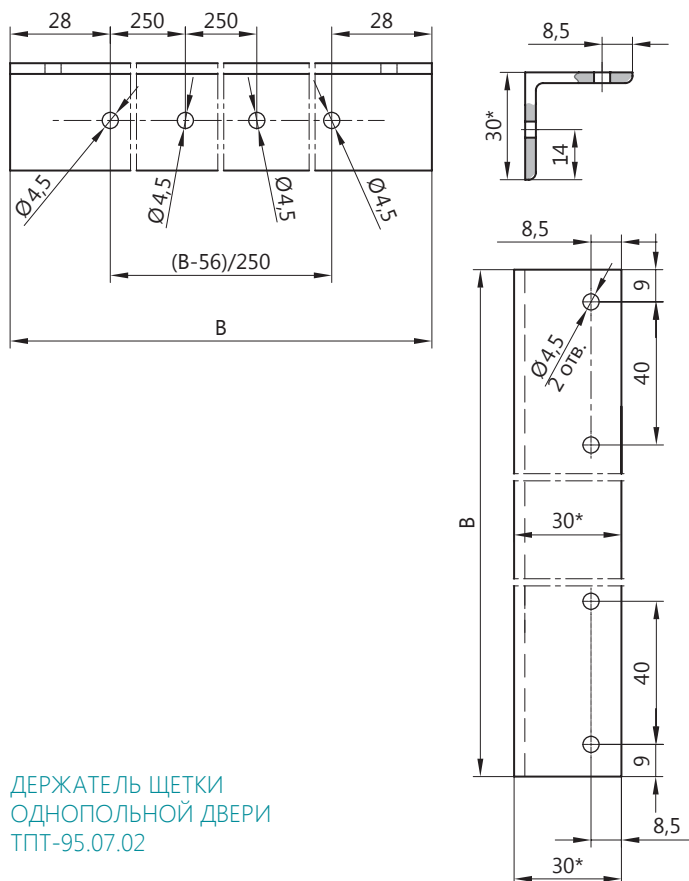
УГОЛОК 30×30×3
