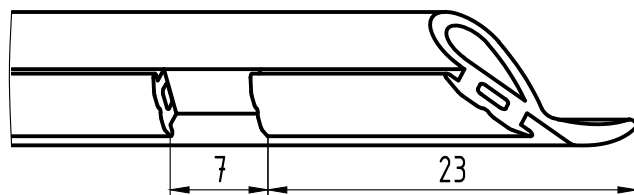
Схема подрезки уплотнителя МПУ-64003
